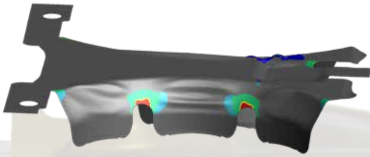
Vorhersage der Risse und Falten mit Stampack
